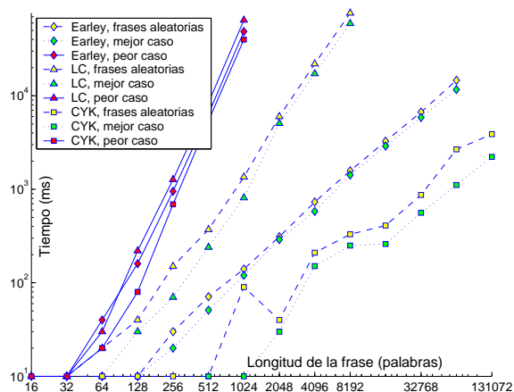
Figura 3: Rendimientos para la gramática de los paréntesis.
